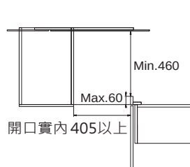
開啟角度與相鄰櫃體示意圖
