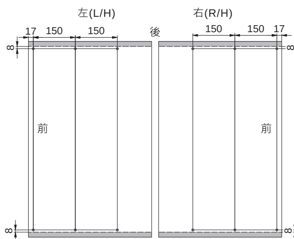
側板尺寸圖
