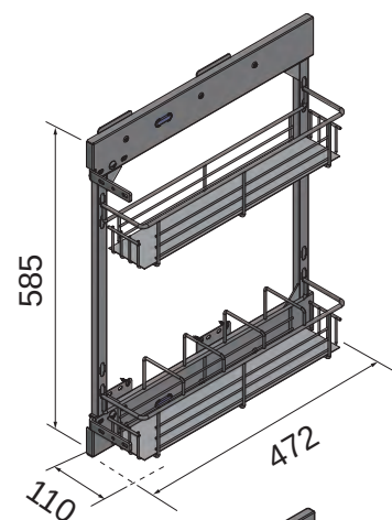
示意圖 Schematic
