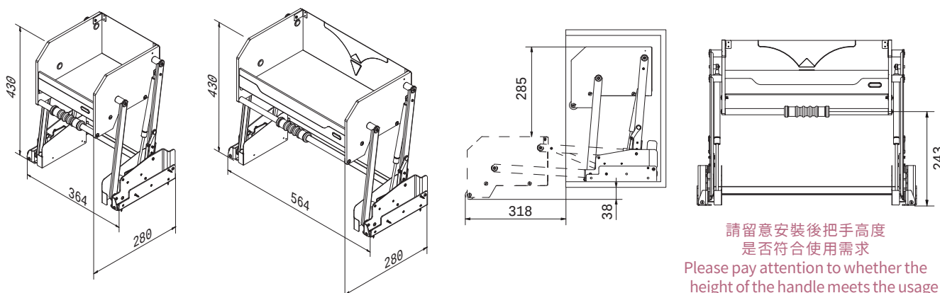
示意圖 Schematic
