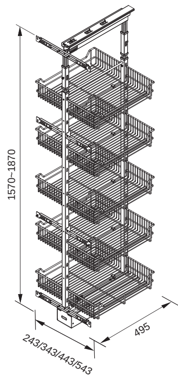
示意圖 Schematic
