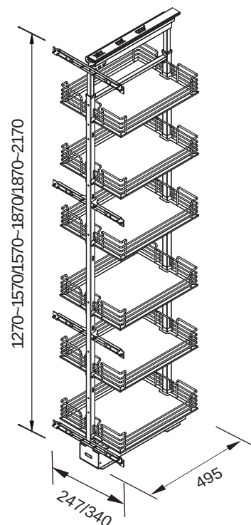
示意圖 Schematic
