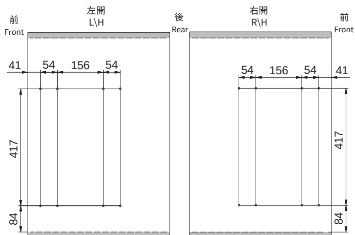
側板孔位示意圖 Side Wall Schematic
