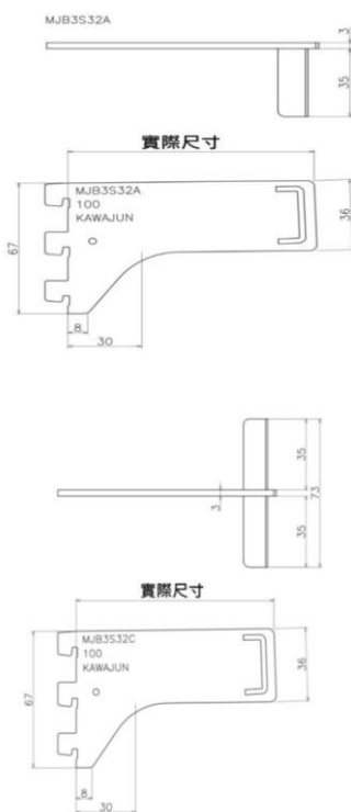
角管用架手
