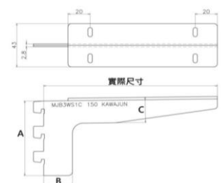
3齒 (中)
