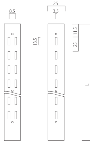
剖面圖
