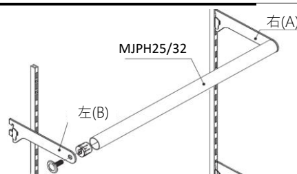
施工範例
