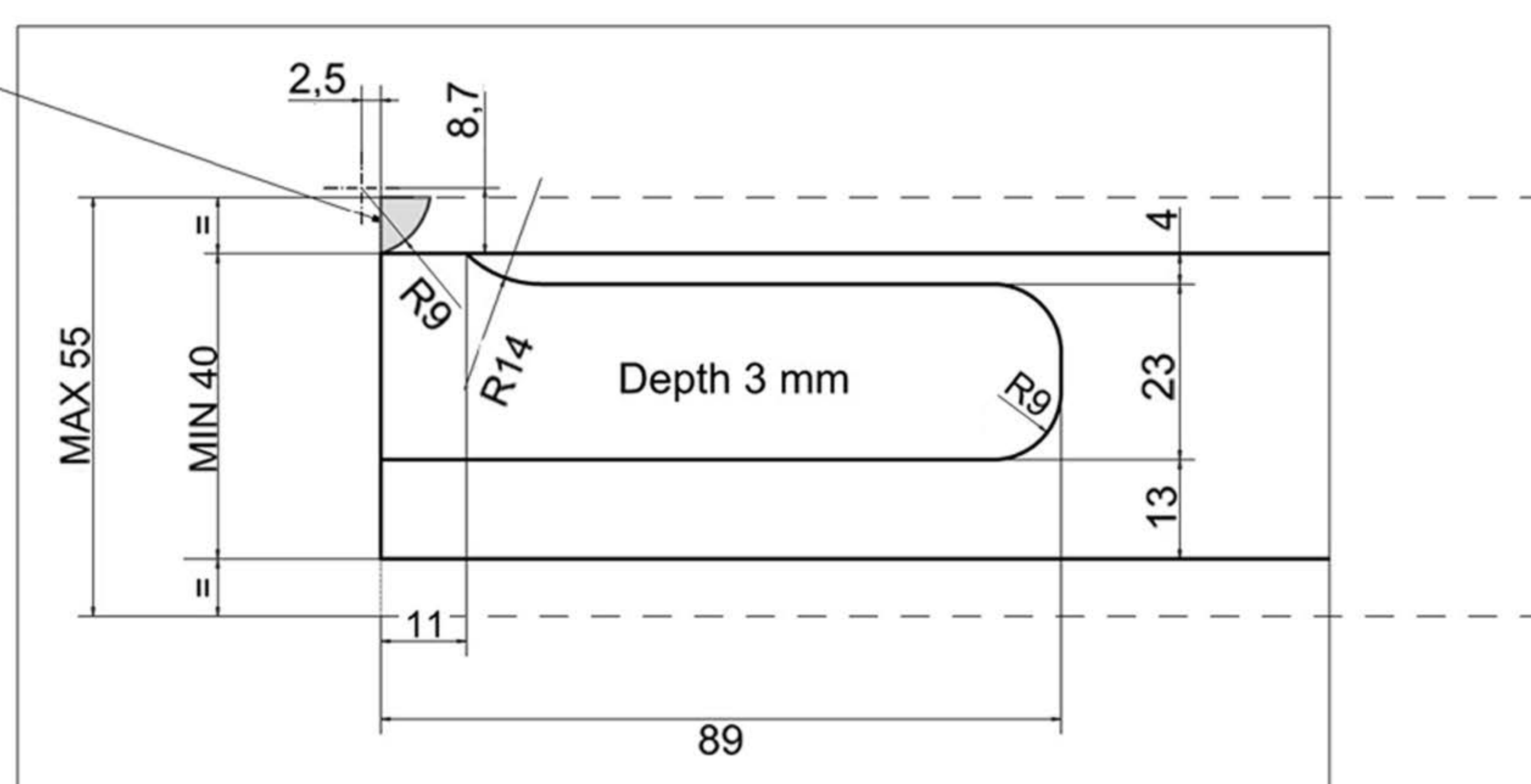
Door Leaf 2
