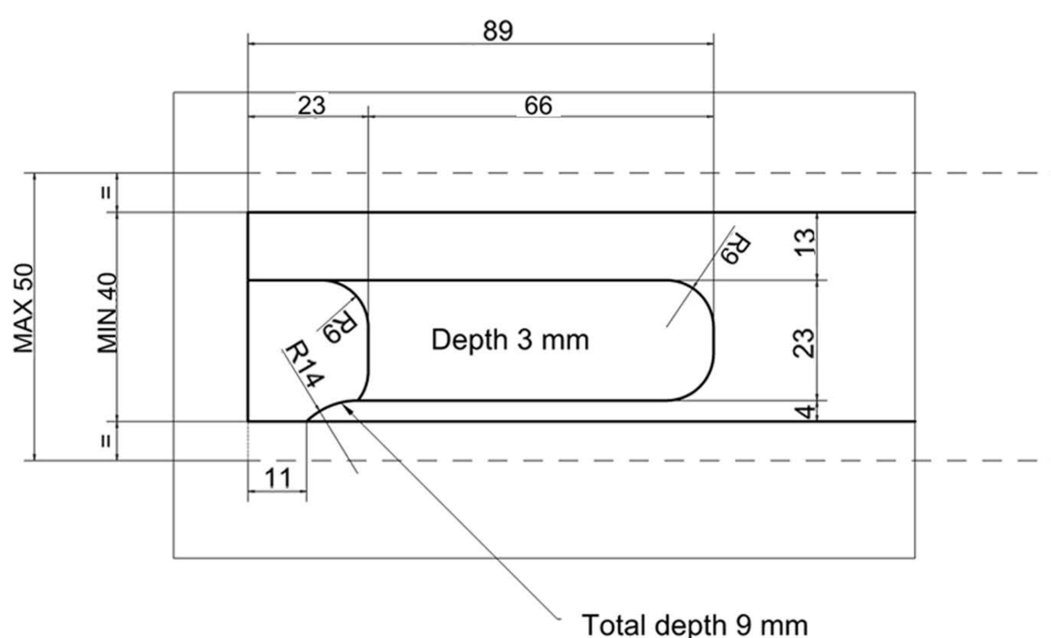
Door Leaf 1
